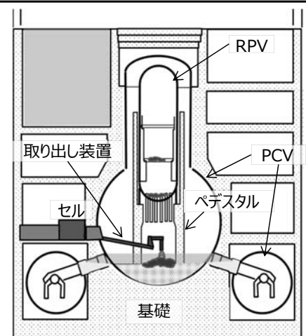
気中－横アクセス工法のイメージ
